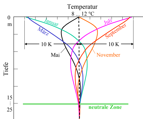
Bild 7.28 Idealisierter Temperaturverlauf im Erdreich
