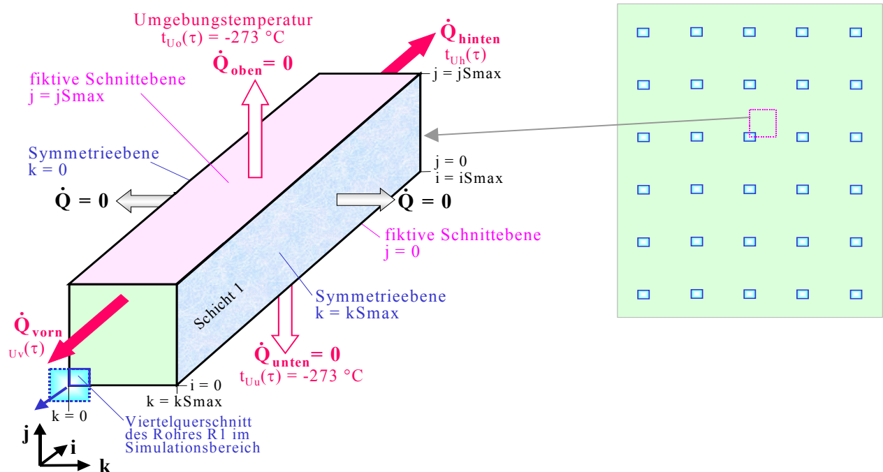
Bild 3.16 Definition eines Minimalausschnittes (links) aus einem Speicherkörper mit Rohrdurchgang (rechts) zur Verkürzung der Simulationszeit Der Simulationsbereich beträgt nur noch ein Viertel des im Bild 3.15 definierten Bereiches.
