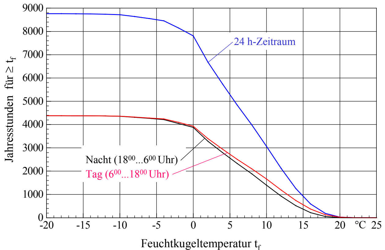
Bild 7.3 Summe der Jahresstunden einer Feuchtkugeltemperatur \geq t_f für drei verschiedene Tageszeiträume entwickelt aus den Daten der DIN 4710 für den Standort Kassel
