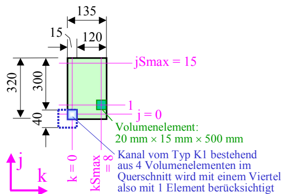
Bild 6.2 Geometrie des Simulationsgebietes für nachfolgende Testbeispiele mit Angaben in mm (nicht maßstäblich) In i-Richtung – in die Tafelebene hinein – gelten die Unterteilungen i = 0 bis i_{\text{Smax}} = 19 , sodass die Länge des Speicherkörpers 10 m beträgt.
