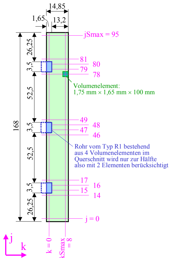
Bild 5.16 Geometrie des Simulationsgebietes für Test 2 mit Angaben in mm (nicht maßstäblich) In i-Richtung – in die Tafelenebene hinein – gelten die Unterteilungen i = 0 bis i_{\text{Smax}} = 19 , sodass die Länge des Speicherkörpers 2000 mm beträgt.
