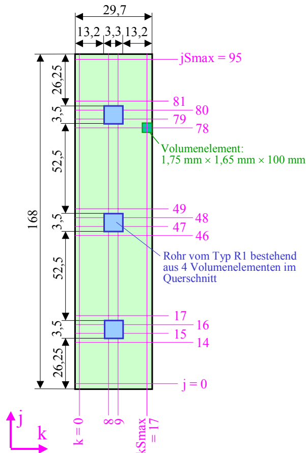
Bild 5.3 Geometrie des Simulationsgebietes für Test 1 mit Angaben in mm (nicht maßstäblich). In i-Richtung – in die Tafelebene hinein – gelten die Unterteilungen i = 0 bis i_{\text{Smax}} = 19 , sodass die Länge des Speicherkörpers 2000 mm beträgt.
