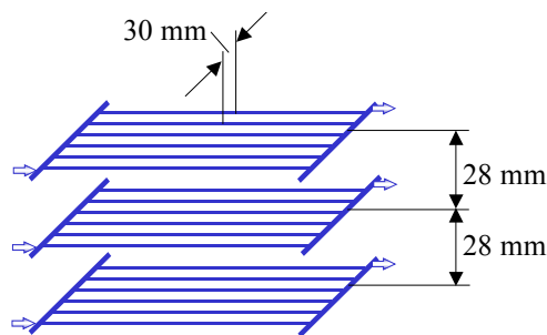
Bild 8.15 Hauptabmessungen für das Rohrregister im Speicherkörper
