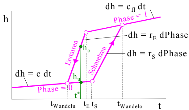
Bild 3.5 Verlauf der spezifischen Enthalpie h(t, \text{Phase}) in Abhängigkeit der Materialtemperatur t und des verlaufsabhängigen Phasenzustandes \text{Phase} bei einer Hysterese nach Form B
