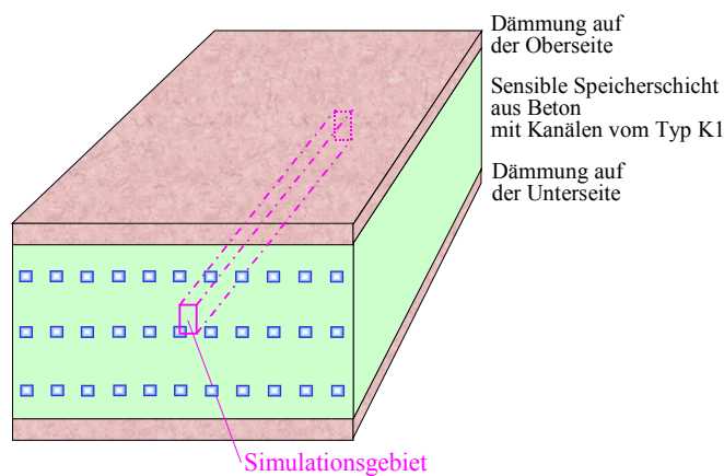
Bild 6.1 Wärmespeicher aus Beton mit Kennzeichnung des Simulationsgebietes für die nachfolgenden Testbeispiele Es wird nur ein Viertel des Luftkanals und ein zugehöriger Symmetriebereich des Speichermaterials einbezogen. Die Dämmschichten an der Ober- und Unterseite bleiben unbeachtet.
